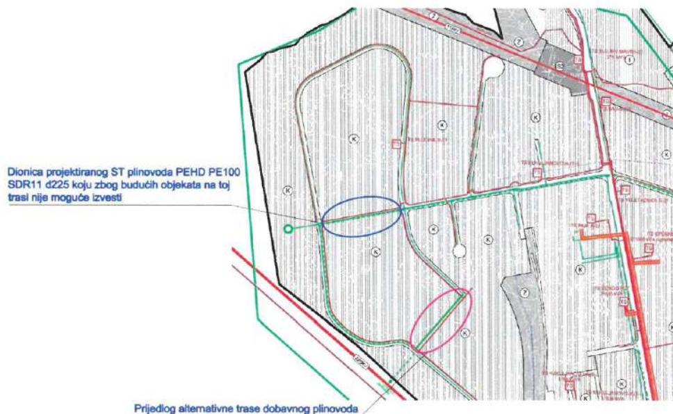
Skica 1. Prijedlog trase alternativnog dobavnog plinovoda
